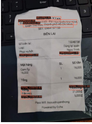
(a) Roi-Pooling
